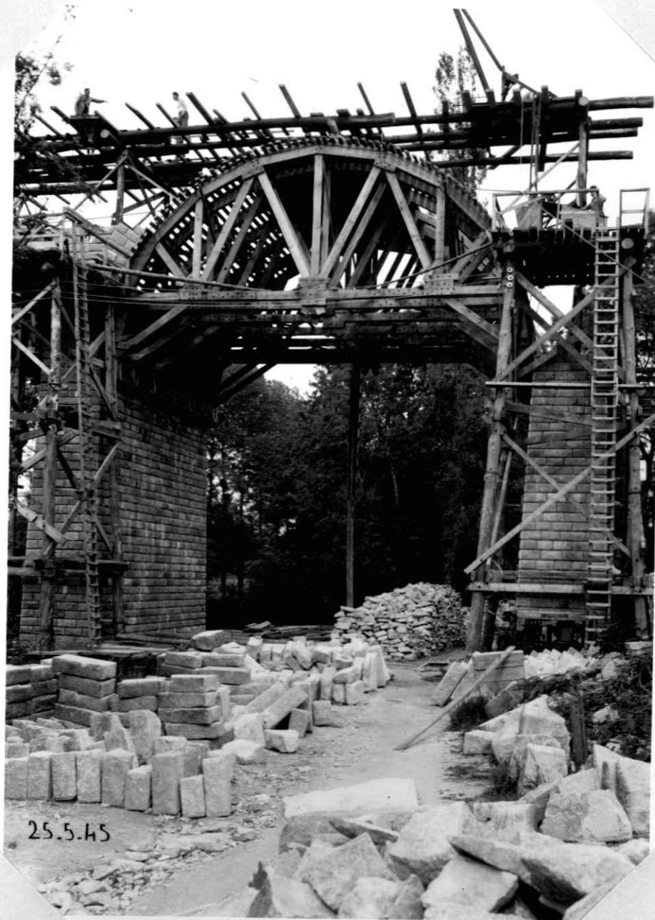
Pont de Montaiqu - Cintre de la 2 ème Voûte
