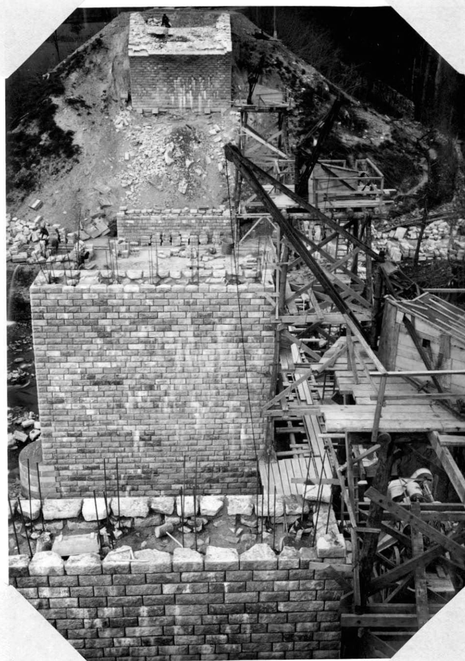
- Maçonnerie des piles - le 27.2.45.
