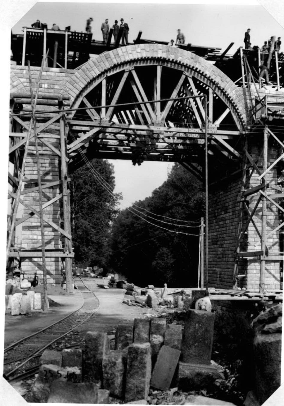
Cintre de la 3 ème Voûte. le 25.5.45
