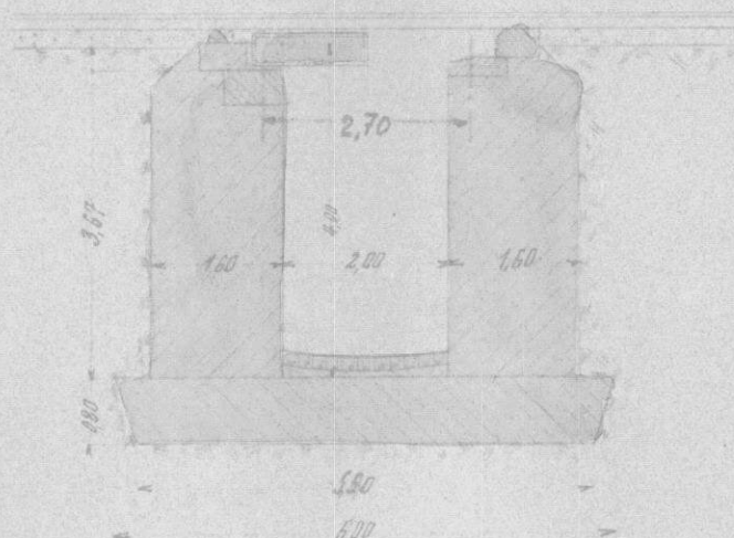
Coupe longitudinale 1:100
