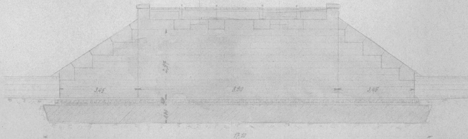
Coupe longitudinale 1:100
