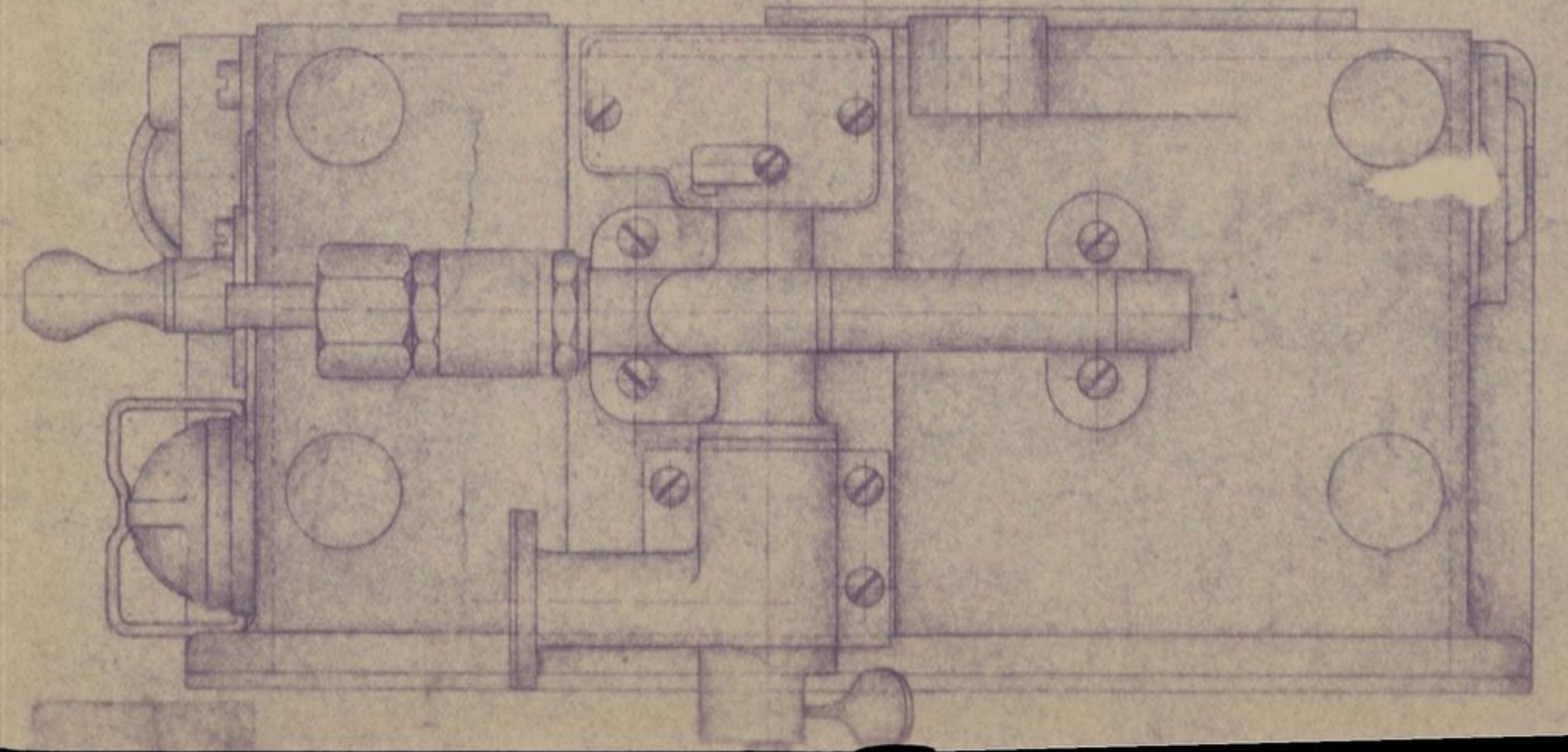
INDICATEUR ENREGISTREUR DE VITESSE SYSTEME FLAMAN AVEC DISPOSITIF D'ENREGISTREMENT ET DE REPETITION DES SIGNAUX
