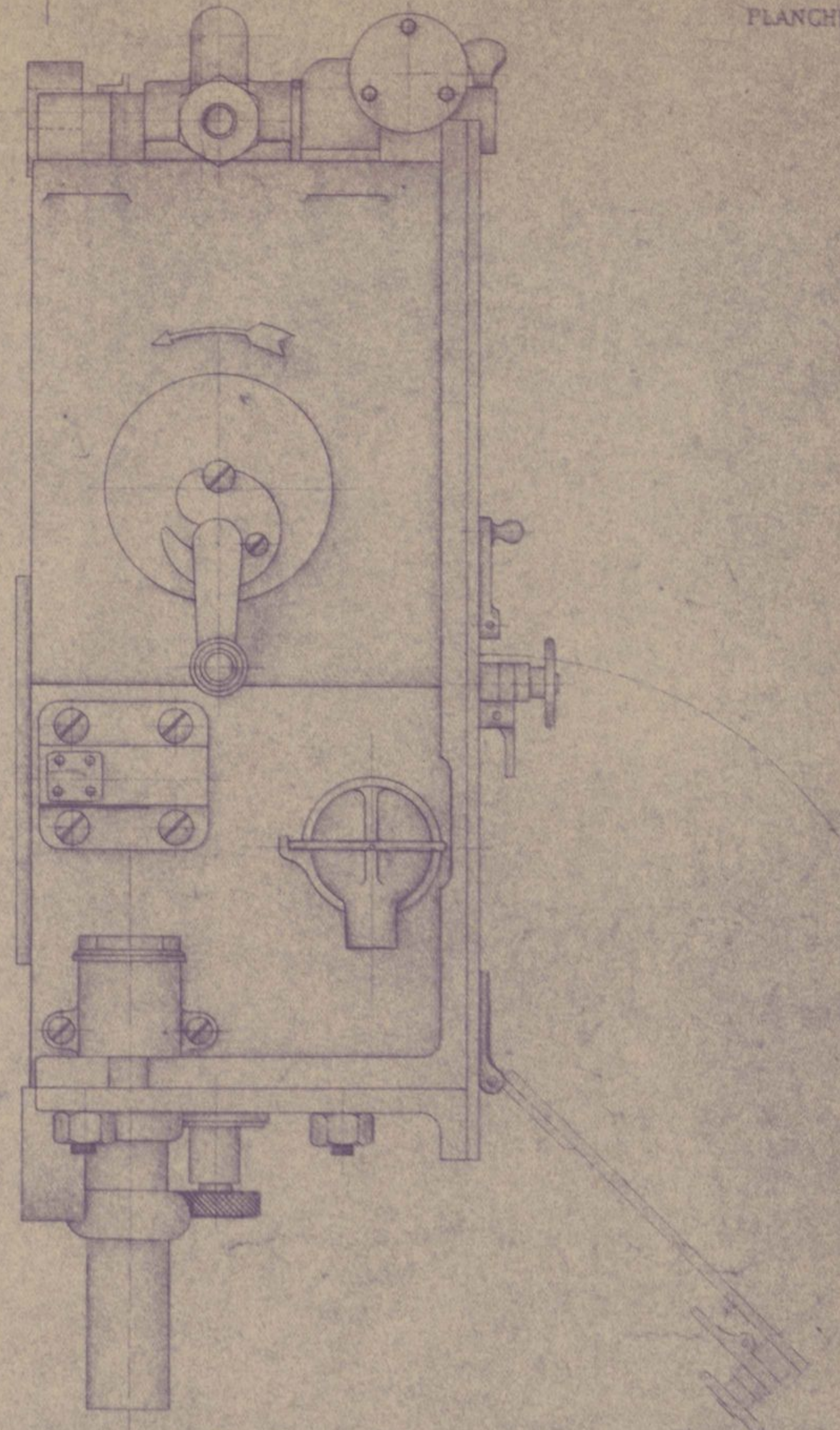
INDICATEUR ENREGISTREUR DE VITESSE SYSTEME FLAMAN AVEC DISPOSITIF D'ENREGISTREMENT ET DE REPETITION DES SIGNAUX
